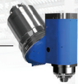
Schwenkfräskopf Dynamisch und hochgenau: Die Fräsköpfe mit Direktantrieb.
